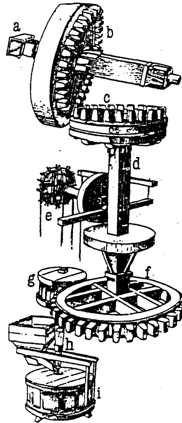
Meccanismo del mulino
